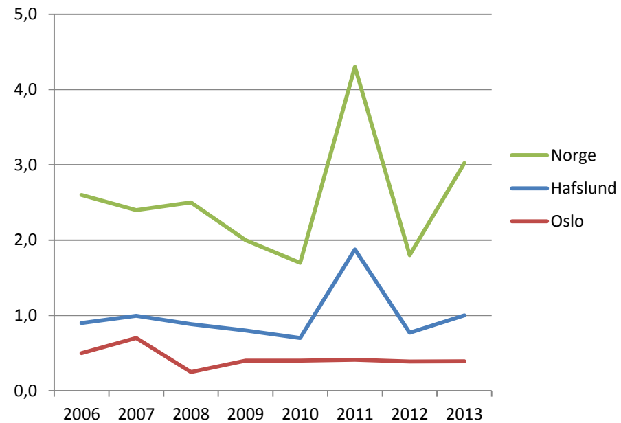
Avbruddenes varighet, SAIDI
